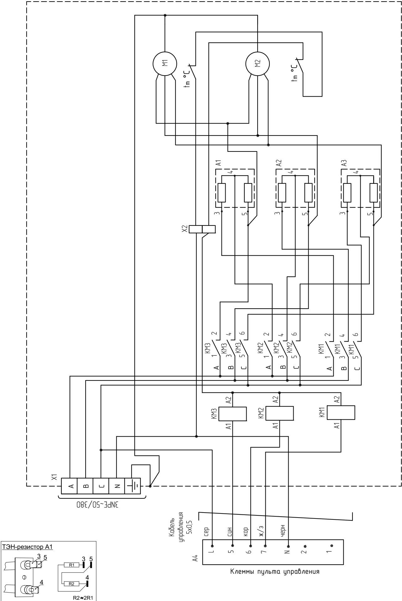
Рисунок 6. Электрическая схема занавесы КЭВ-П5050А
