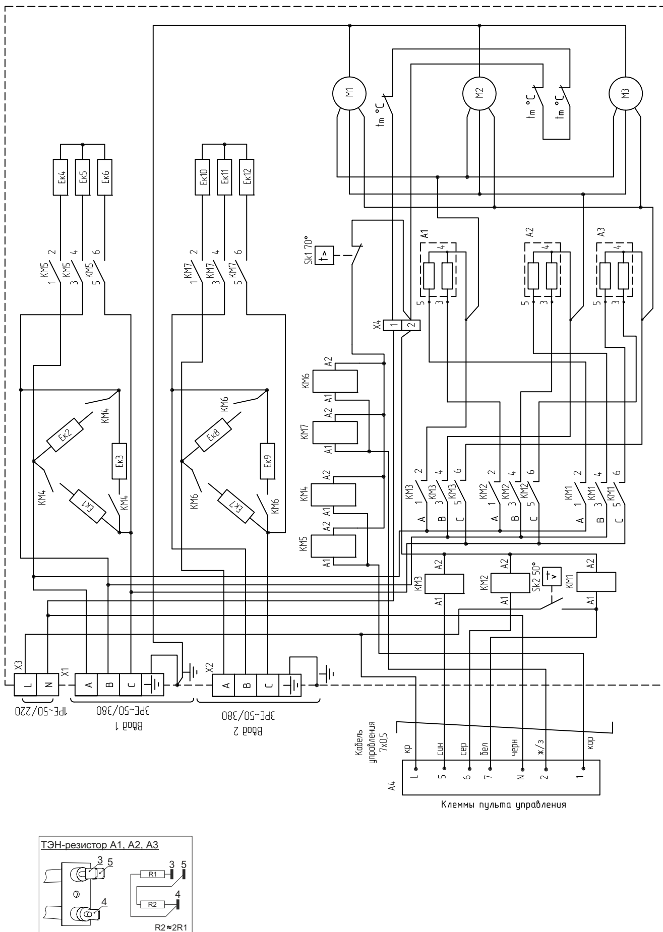
Рисунок 10. Электрическая схема завес КЭВ-48П5060Е
