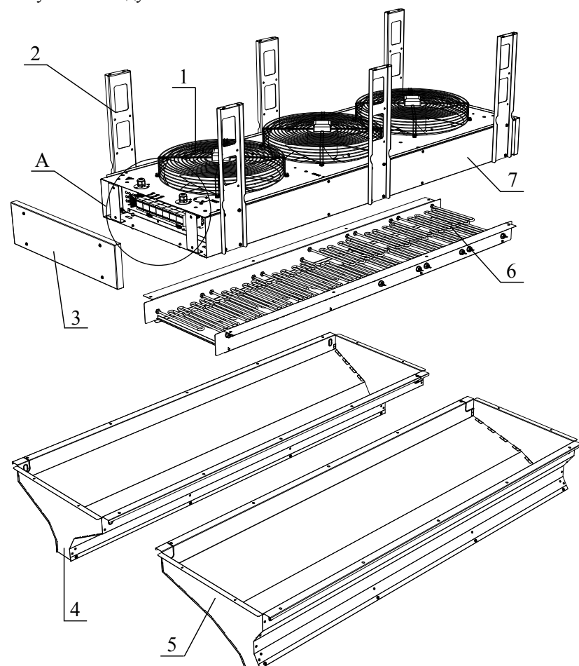
Рисунок 1. Воздушно-тепловая завеса
