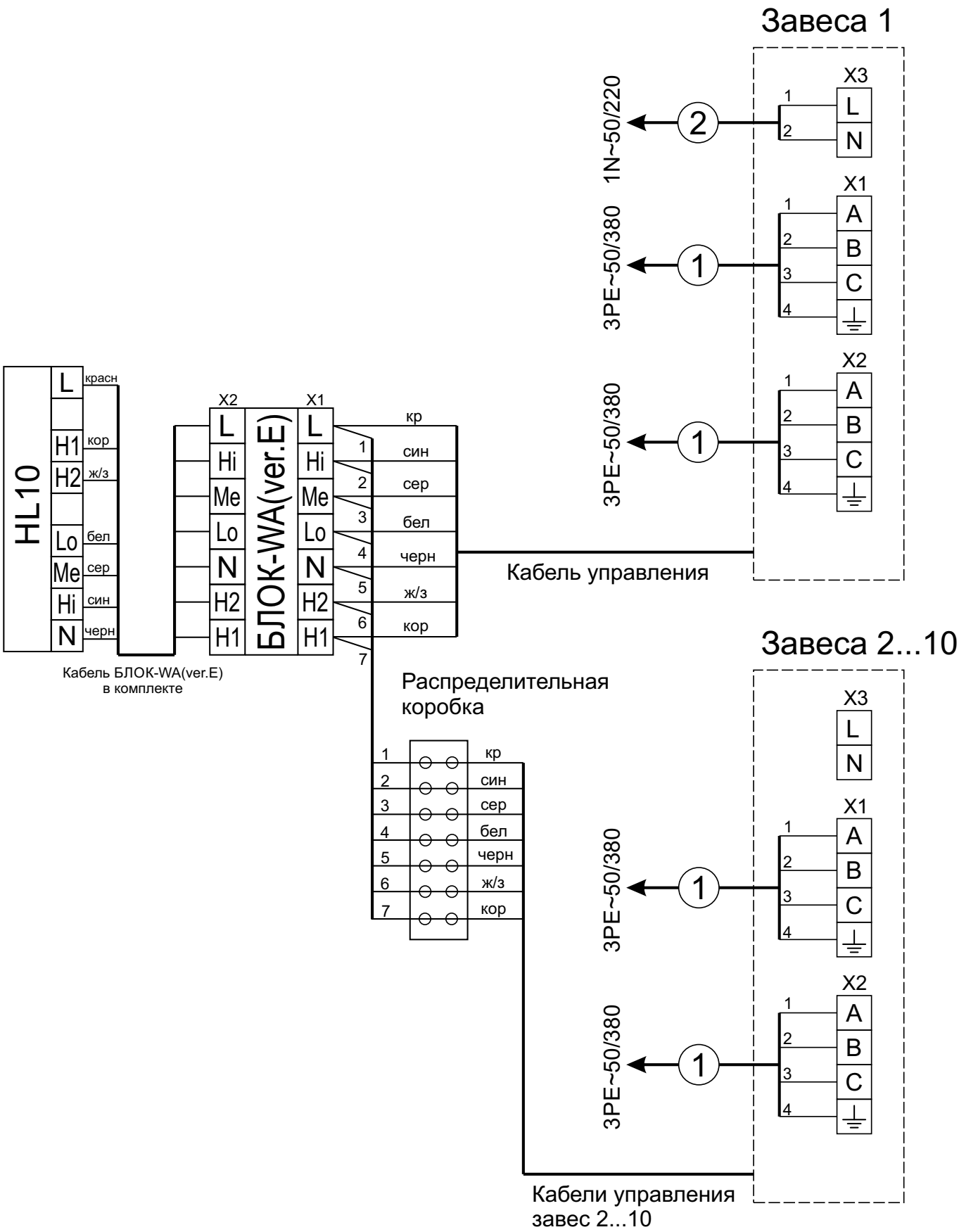
Рисунок 5. Схема подключения от двух до десяти завес к одному пульту управления HL10 через БЛОК-WA(ver.E).
