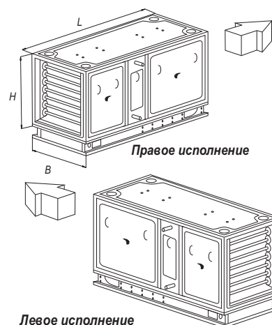
Центральный кондиционер VKC-1,6 с панелями из стали с полимерным покрытием
